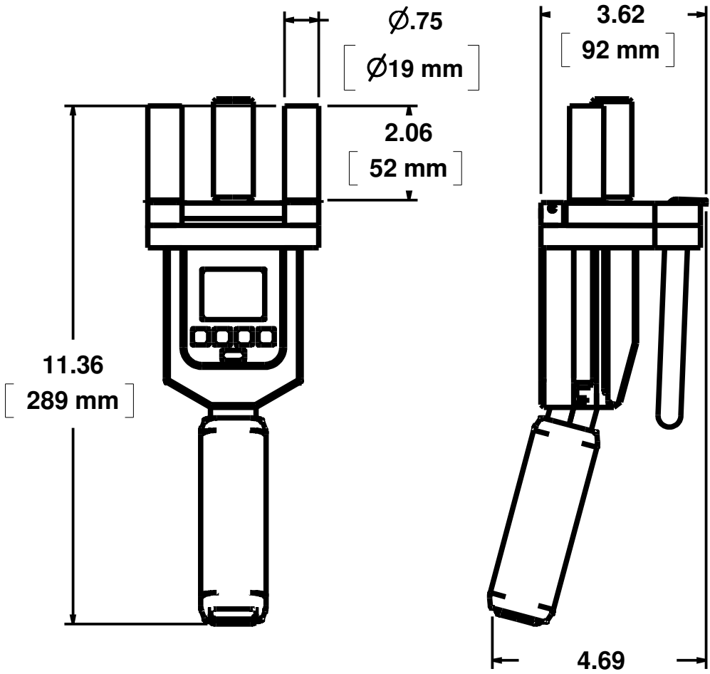
BTX-1 DIGITAL WEB TENSION METER
